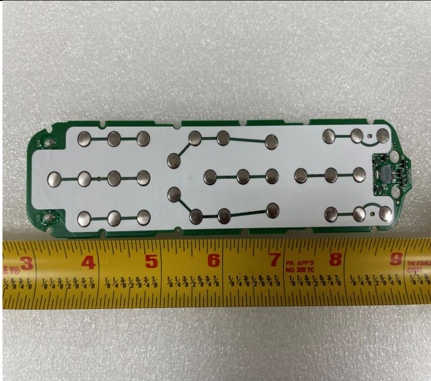
EUT Internal-Front
