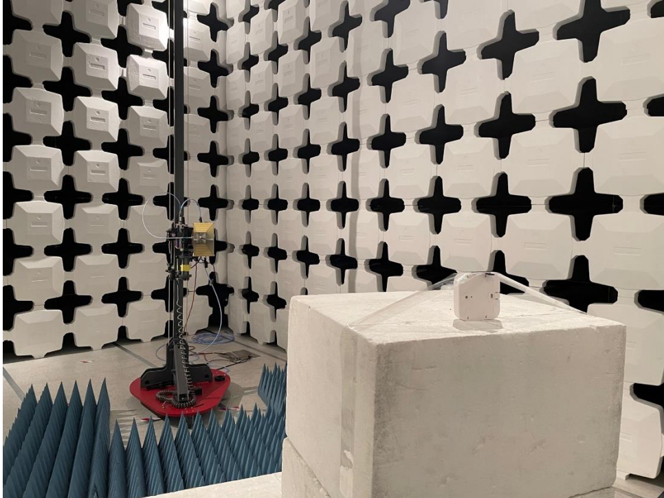
18 GHz -25 GHz
