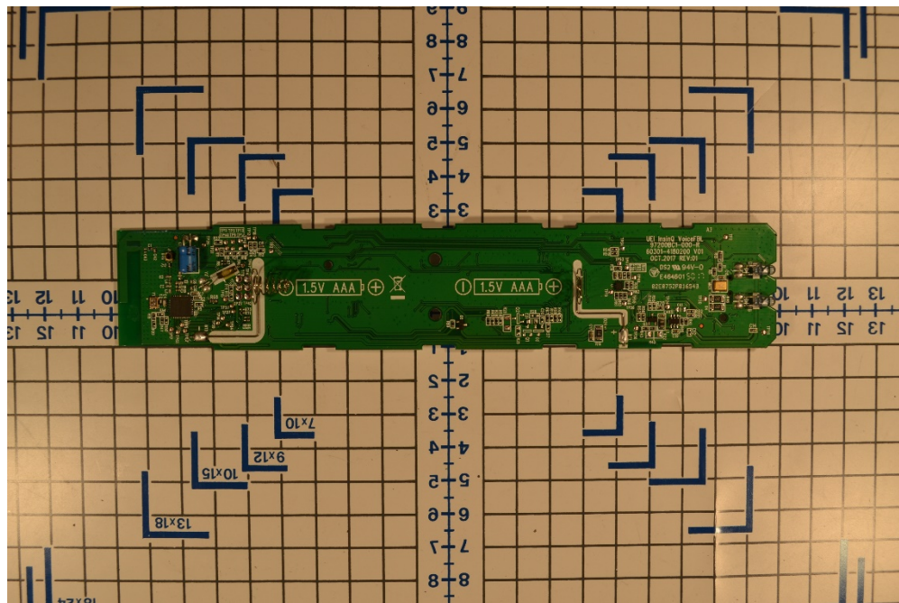
PCB Bottom
