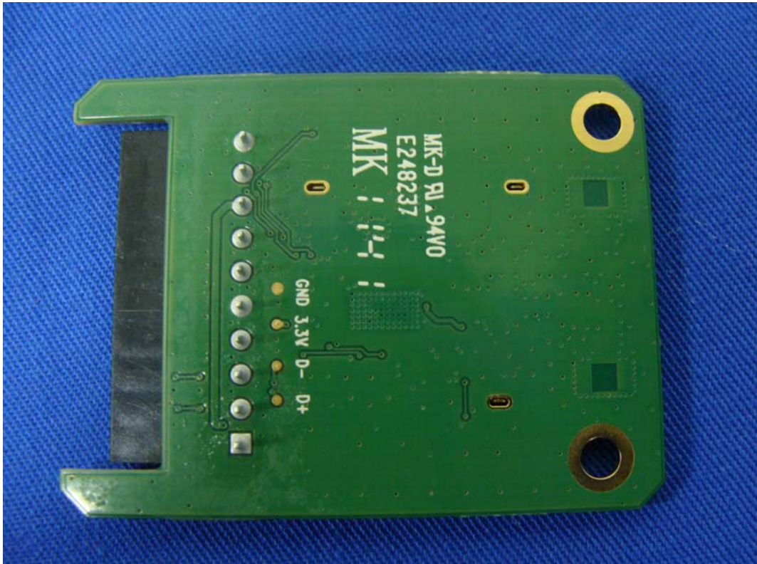
(2) EUT Photo
