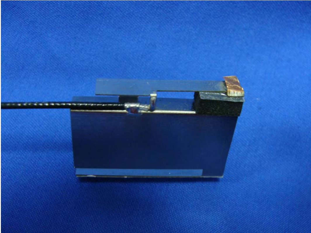
(10) EUT Photo (Antenna-MSA-3415-25GC4-A1)
