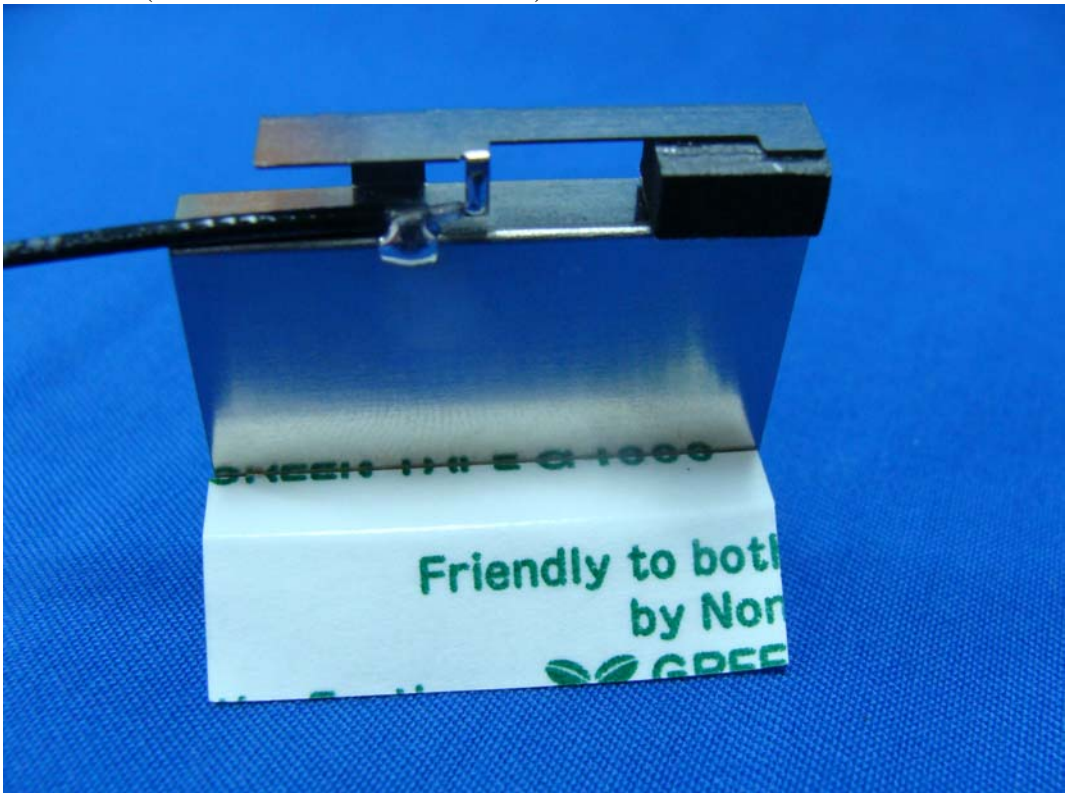
(6) EUT Photo (Antenna-MSA-3422-25GC4-A2)
