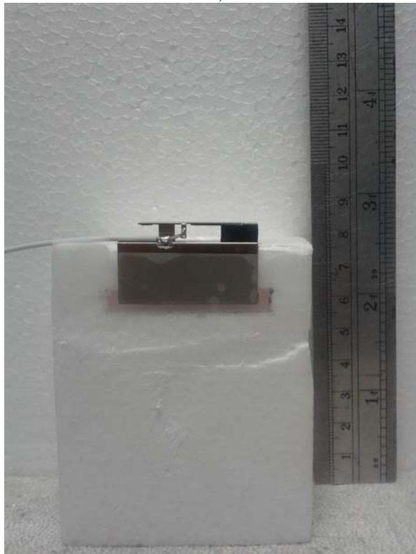
(12) EUT Photo(Antenna-MSA-3415-25GC4-A3)
