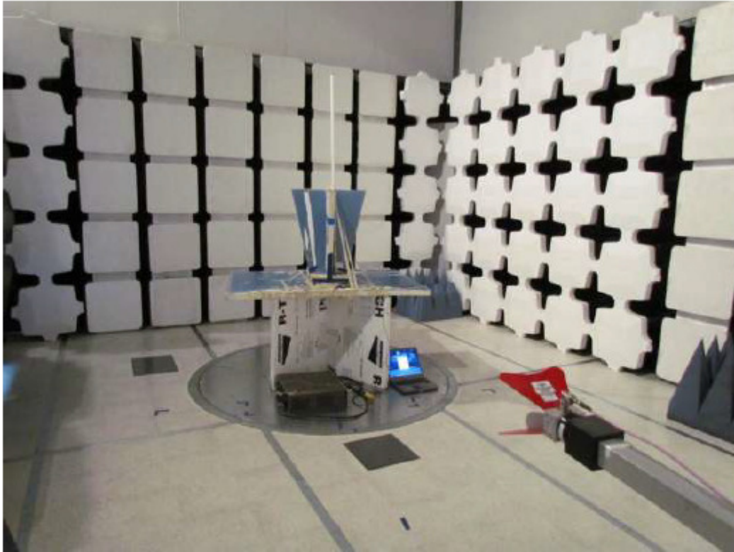
8.1 dBi OMNI antenna
