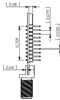
RPSMA
