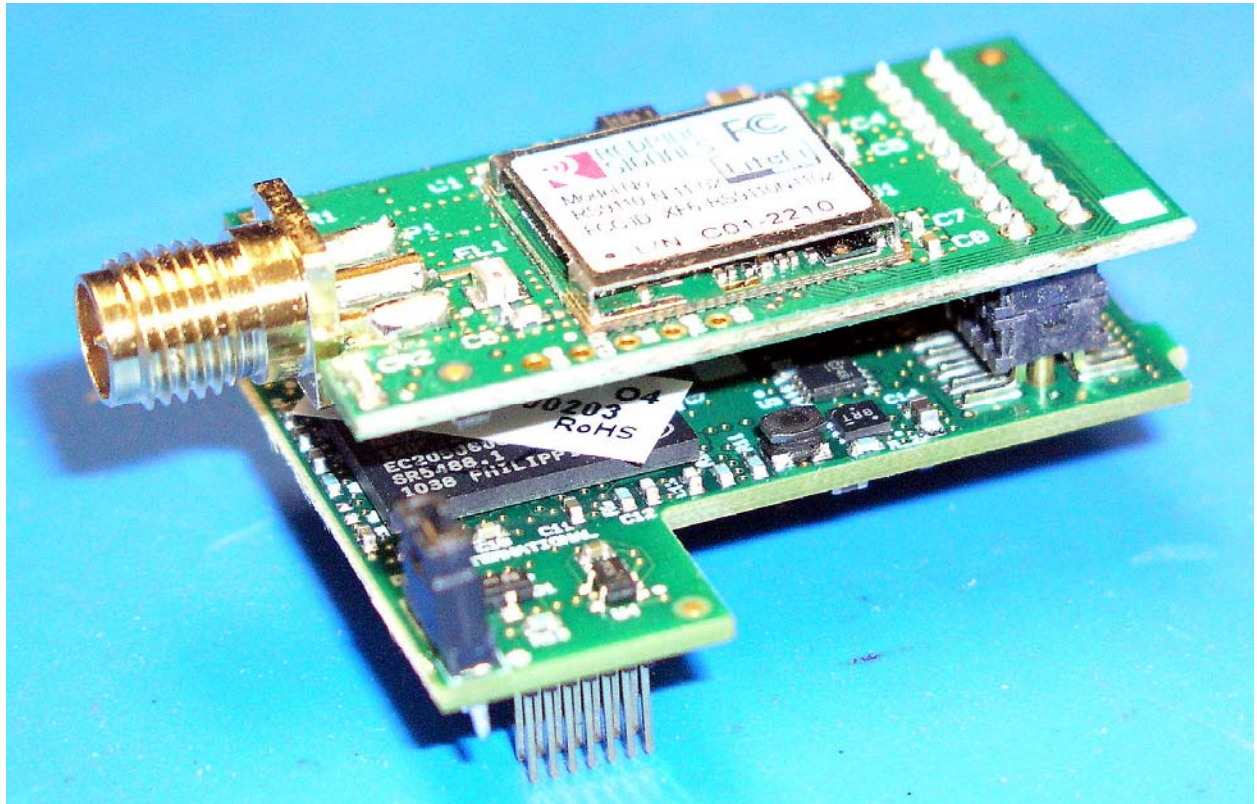
Wi-ME JTAG PCB Stack
