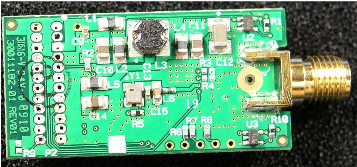
Wi-ME RF PCB Bottom
