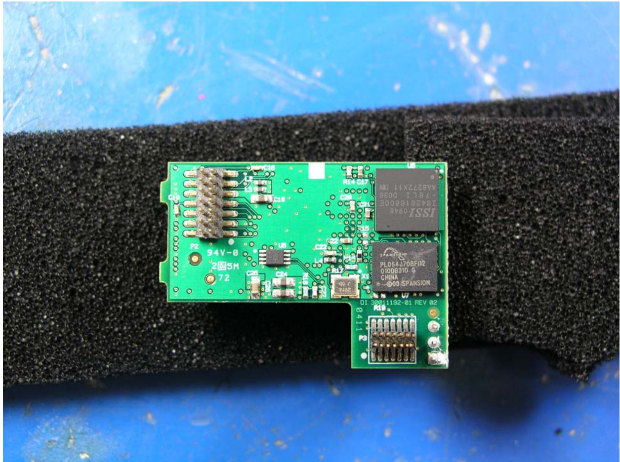
W-Me JTAG PCB Bottom
