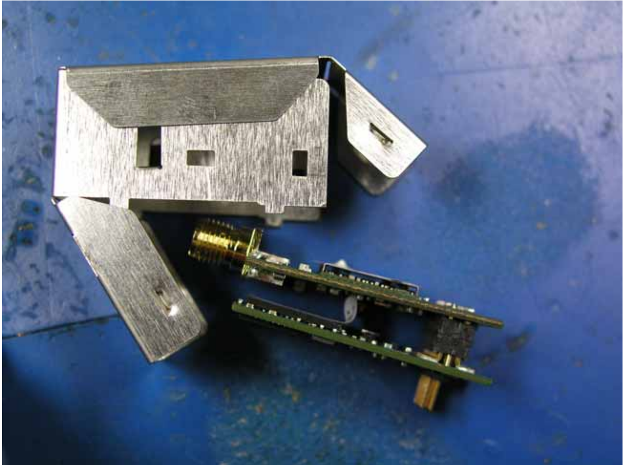
Wi-ME NON JTAG PCB Stack & Enclosure
