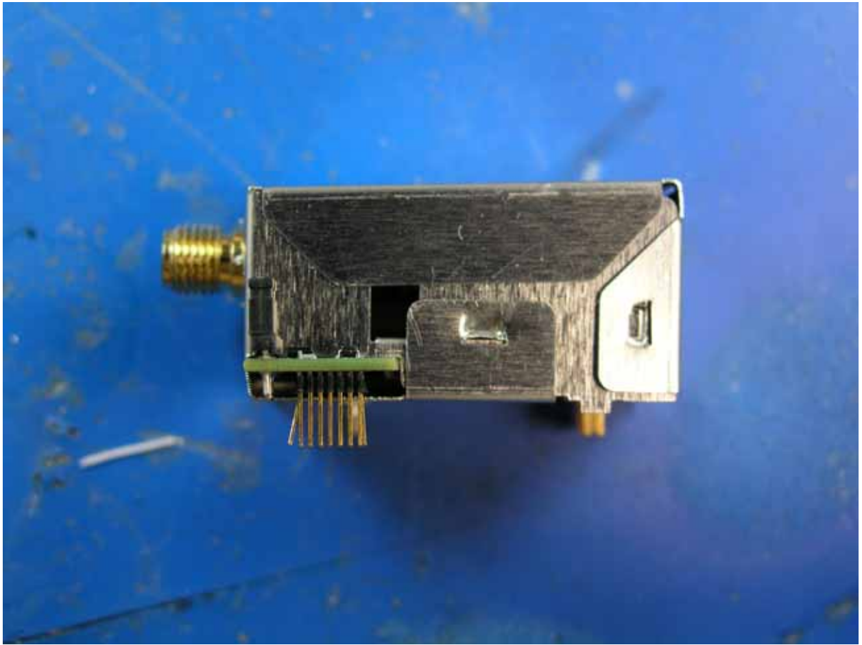
Wi-ME JTAG Side View
