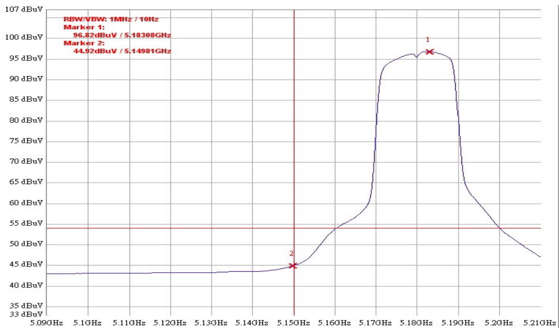
Dual Tx 802.11n (HT20) CH36 AV
