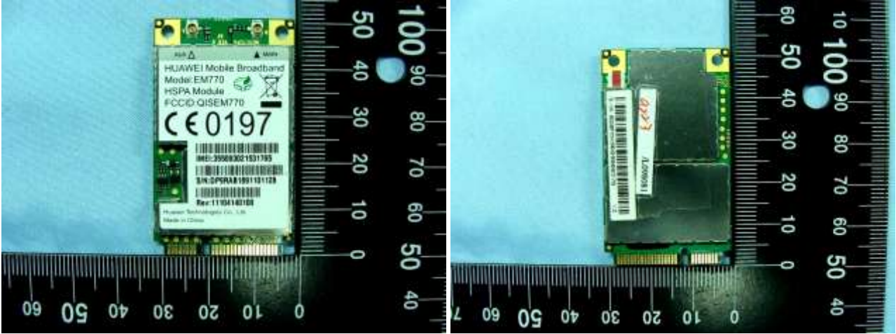
DUT: 3G module (GETAC / EM770)
