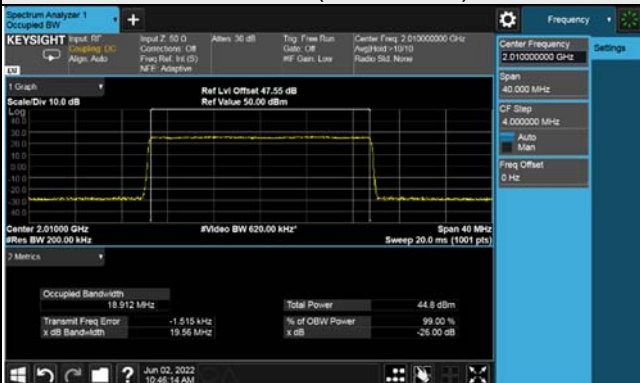
Ch 402000 (2010.0MHz)
