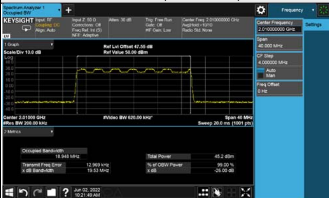
Ch 402000 (2010.0MHz)
