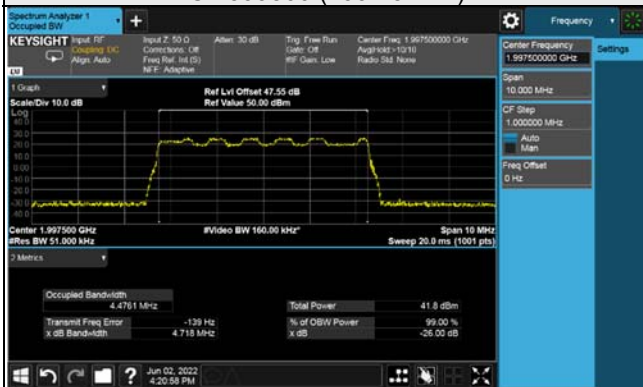
Ch 399500 (1997.5MHz)
