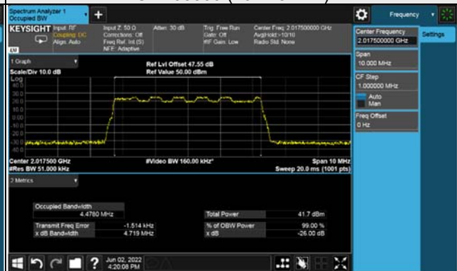
Ch 403500 (2017.5MHz)
