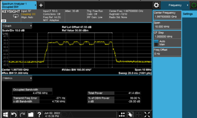
Ch 399500 (1997.5MHz)
