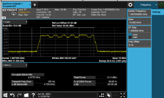
Ch 399500 (1997.5MHz)
