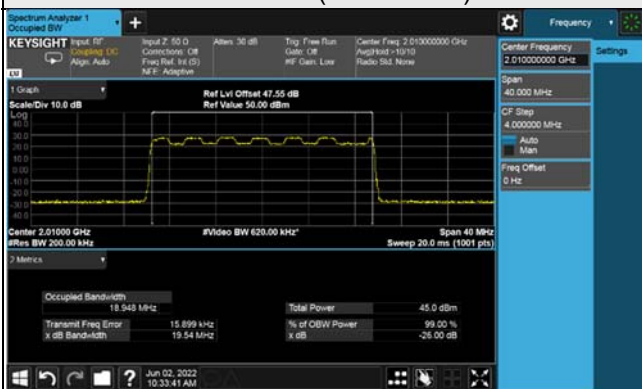
Ch 402000 (2010.0MHz)
