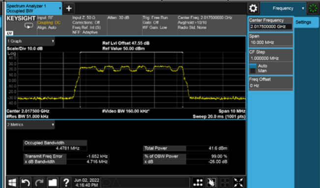
Ch 403500 (2017.5MHz)
