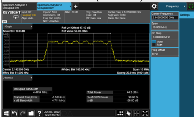
Ch 428500 (2142.5MHz)
