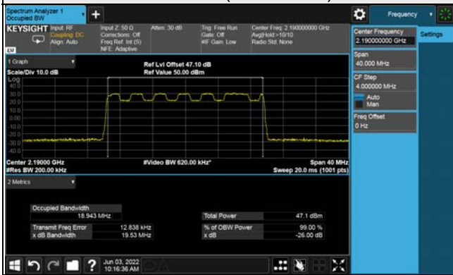
Ch 438000 (2190.0MHz)
