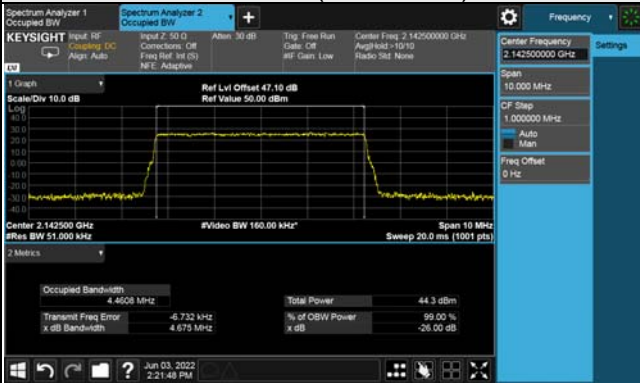
Ch 428500 (2142.5MHz)
