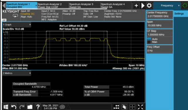
Ch 403500 (2017.5MHz)
