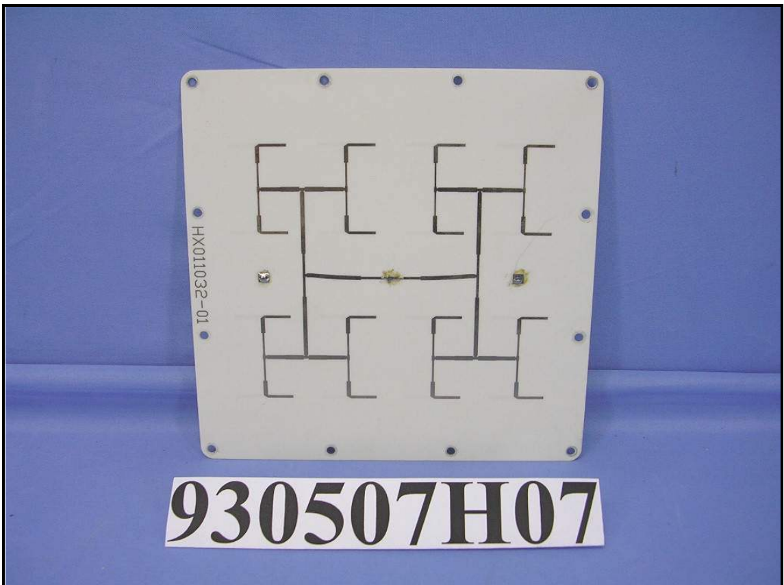
(Antenna 1 – 5GHz)
