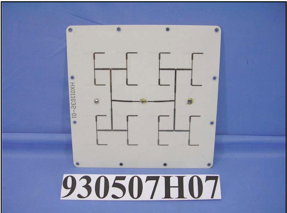
(Antenna 1 – 5GHz)
