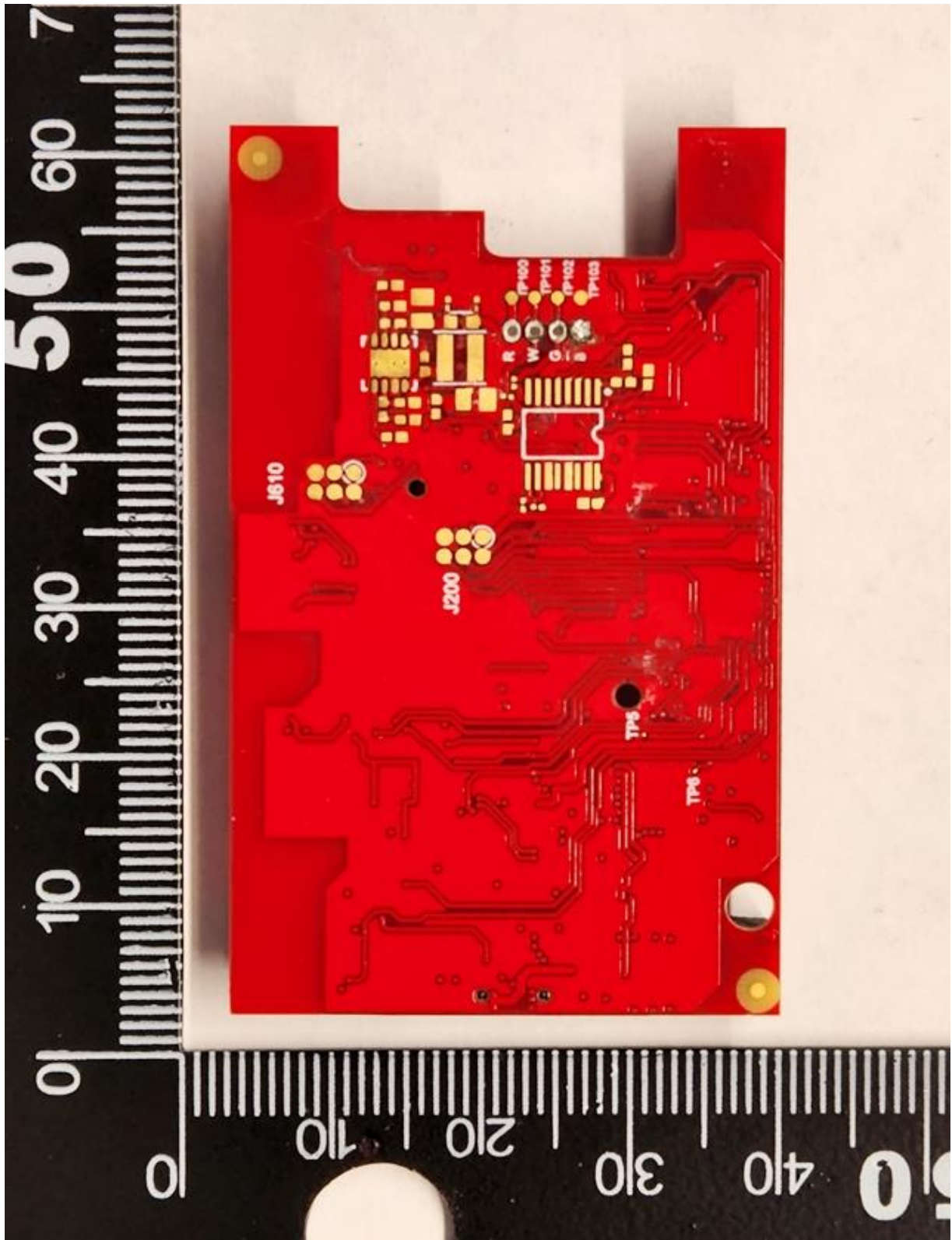
PCB -Bottom
