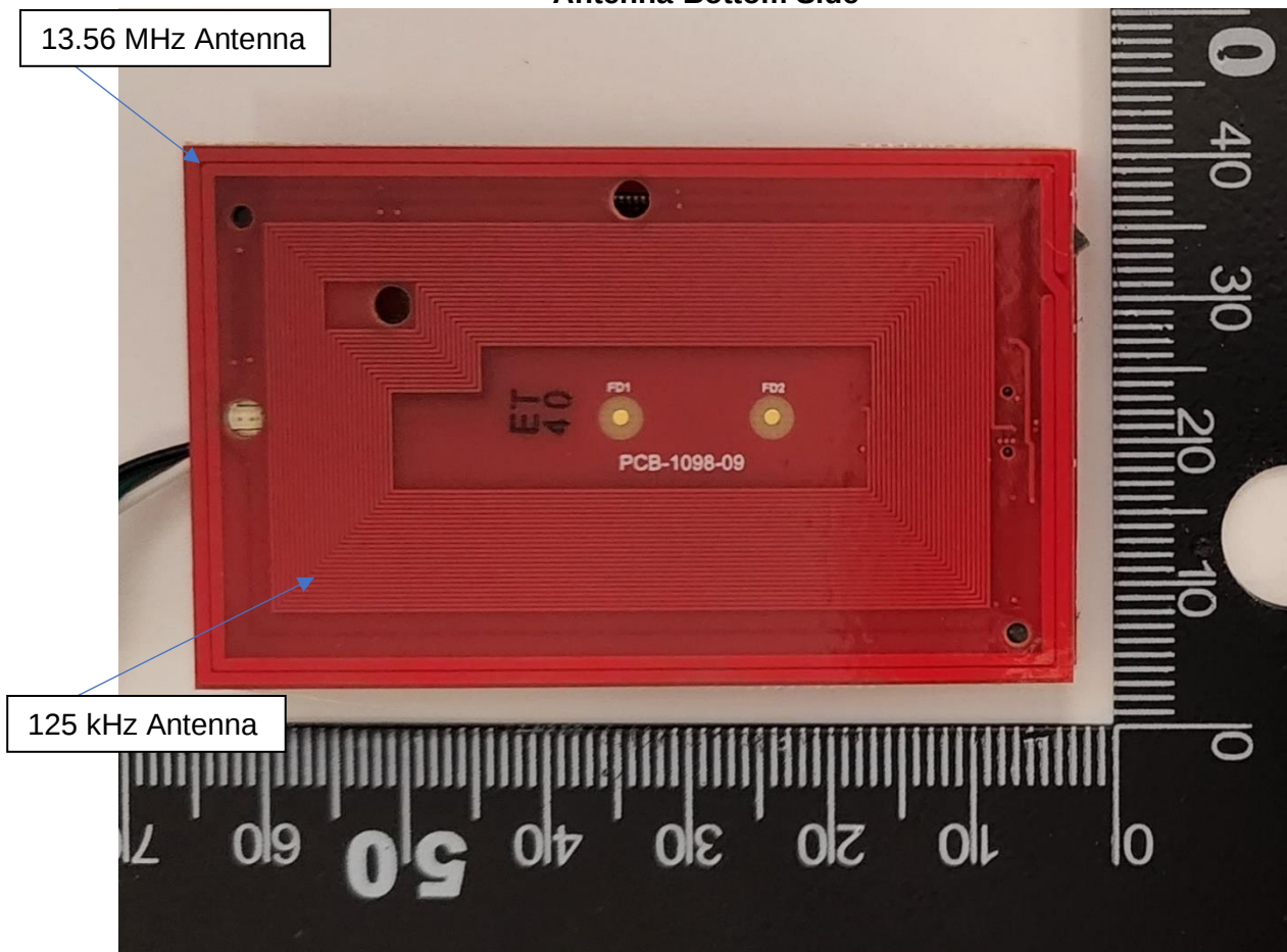
Antenna-Bottom Side
