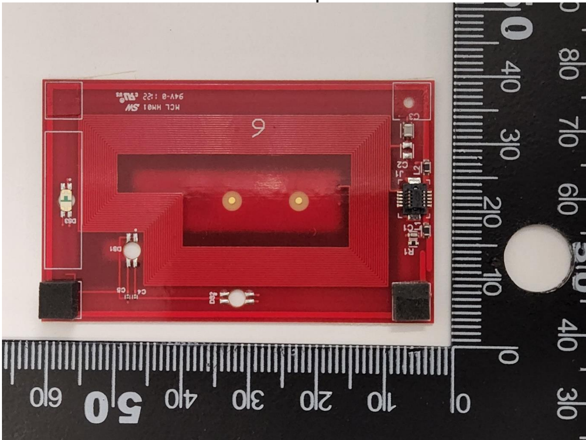
Antenna-Bottom Side
