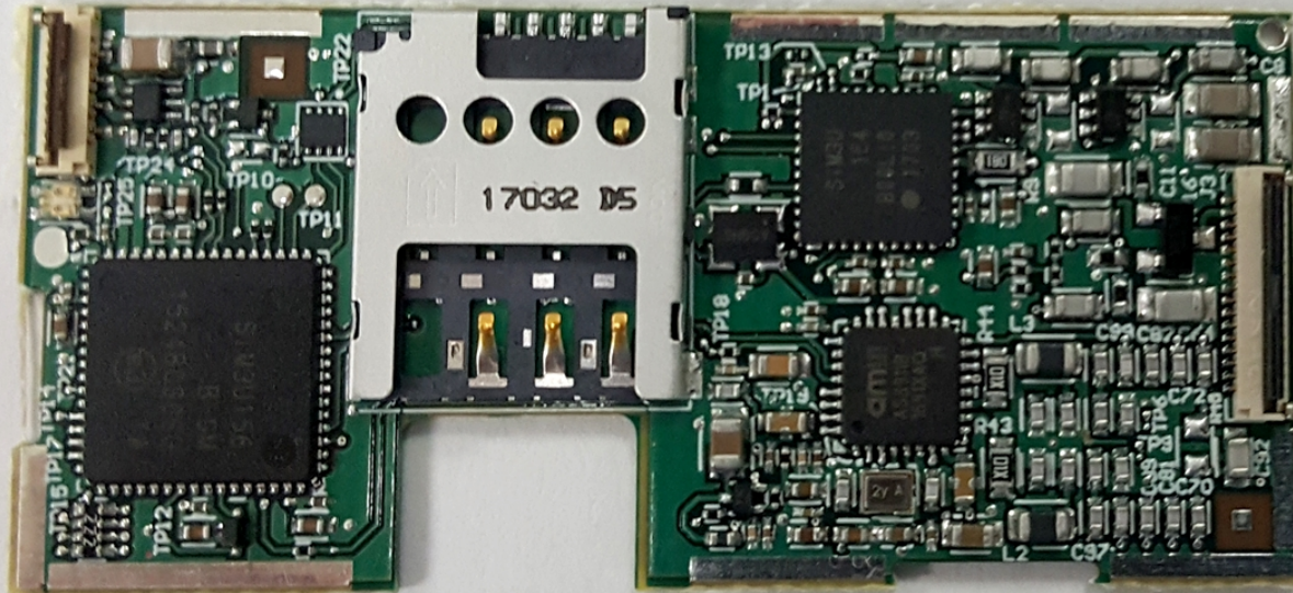
PCB-1066-0A_Top
