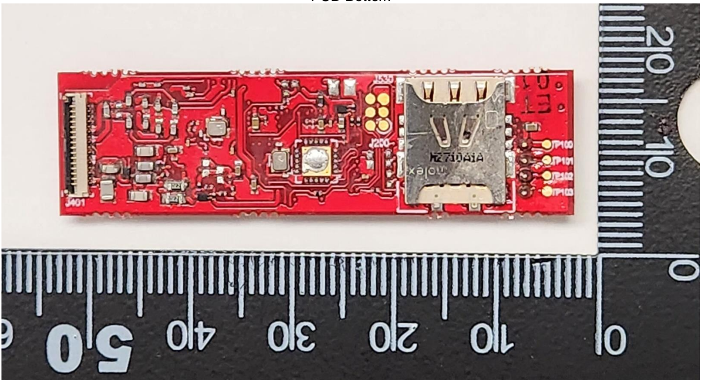
PCB-Bottom
