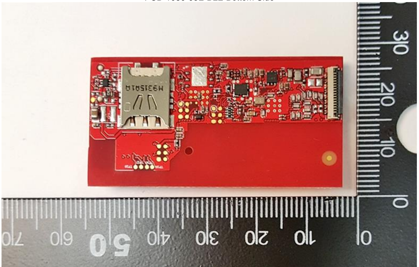
PCB-1080-03E BLE Bottom Side
