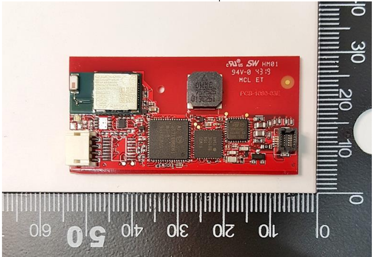
PCB-1080-03E BLE Bottom Side
