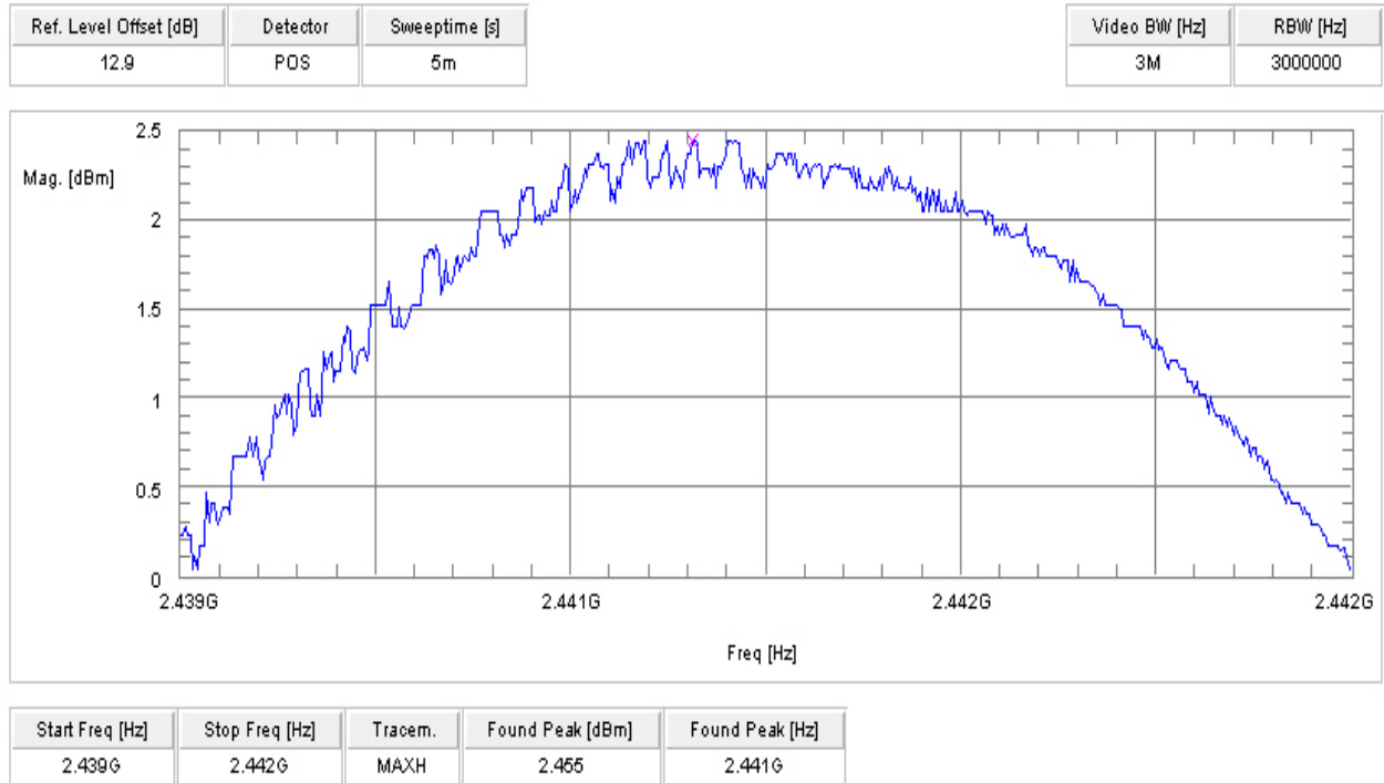
Plot 5 Pi/4 DQPSK
