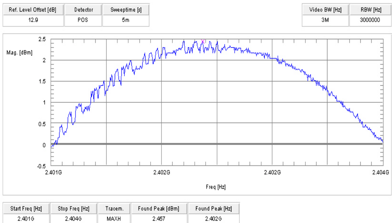
Plot 4 Pi/4 DQPSK
