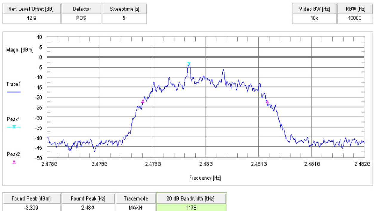
Plot 6 Pi/4 DQPSK
