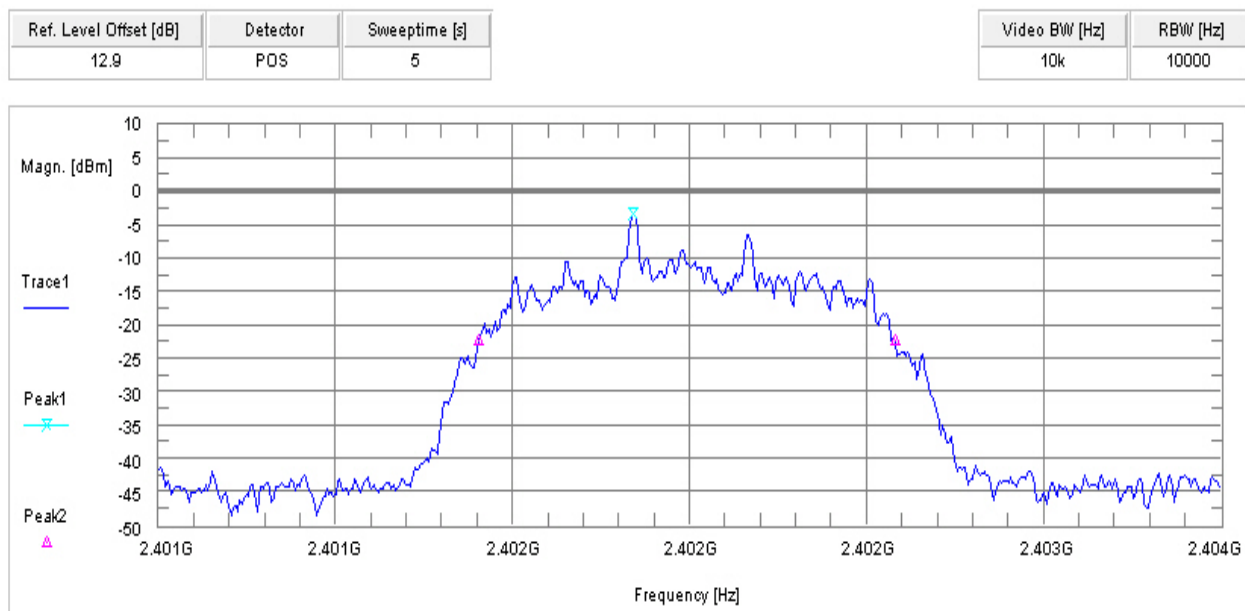
Plot 4 Pi/4 DQPSK
