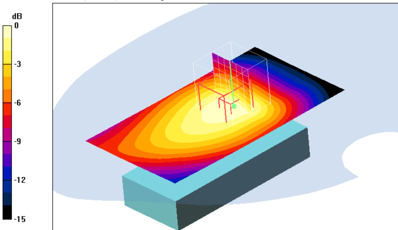
0 dB = 0.466mW/g
