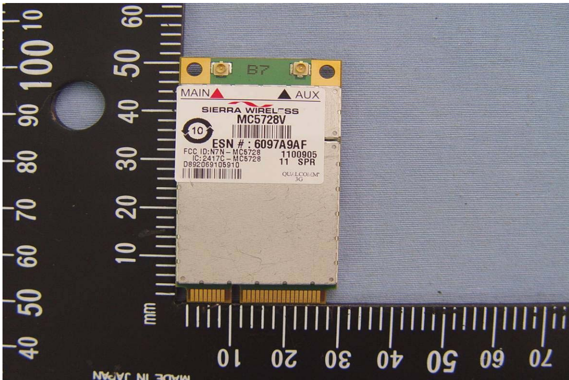
CDMA2000 Module
