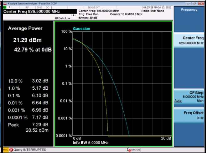
16QAM-20625
