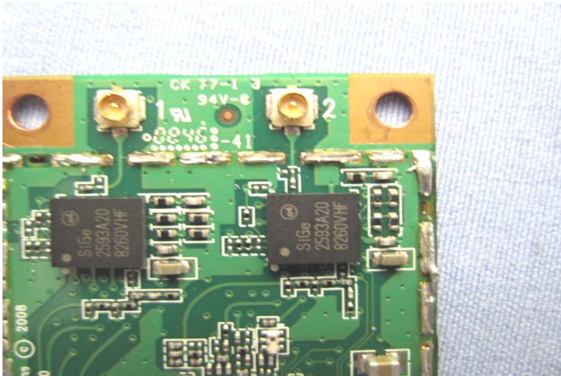
Bluetooth Module
