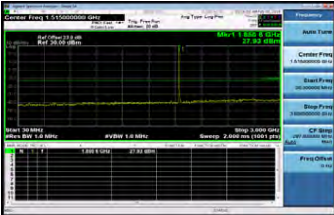
30MHz~3GHz_Band2_3MHz_QPSK_1_0_LowCH18615-1851.5
