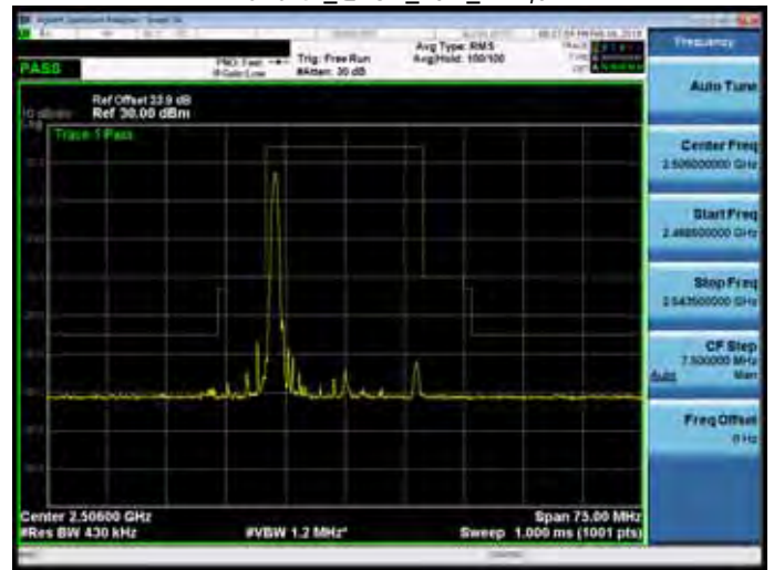
Band 41_QPSK_20M_RB1,99
