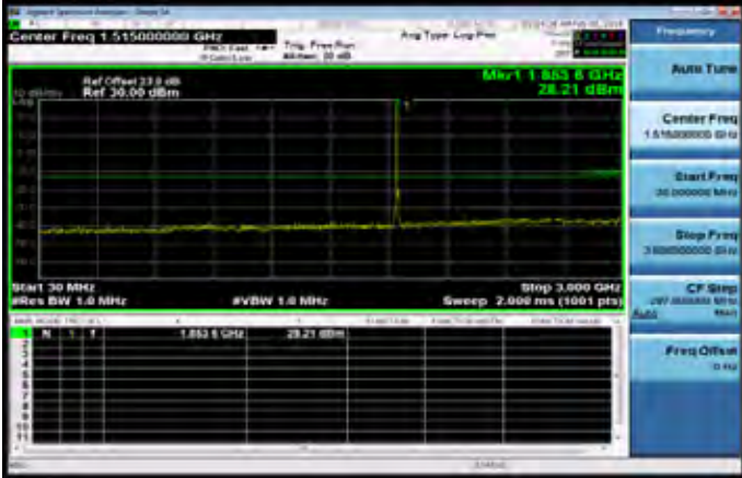
30MHz-3GHz_Band2_10MHz_QPSK_1_0_LowCH18650-1855
