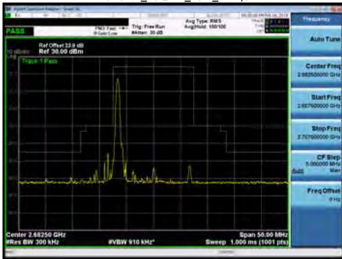
Band 41_16QAM_15M_RB1,74
