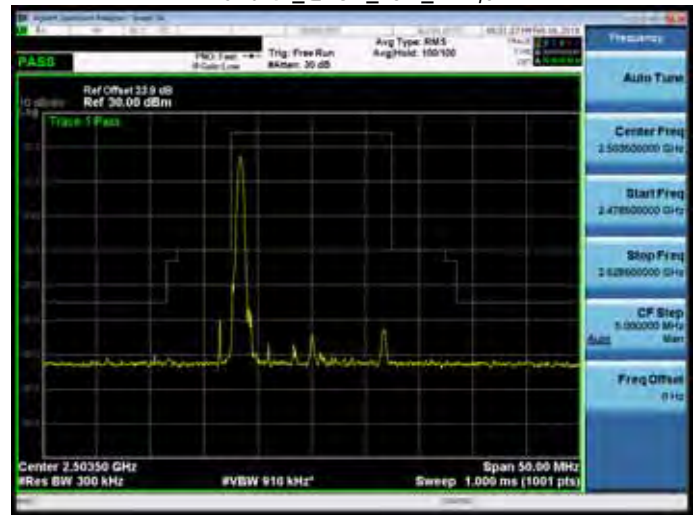
Band 41_QPSK_15M_RB1,74
