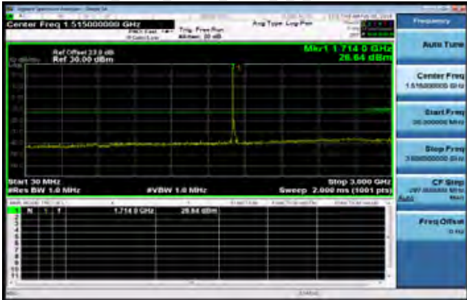
30MHz-3GHz_Band4_20MHz_QPSK_1_0_LowCH20050-1720
