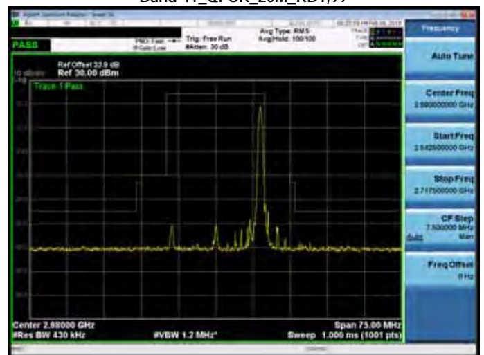
Band 41_QPSK_20M_RB1,99
