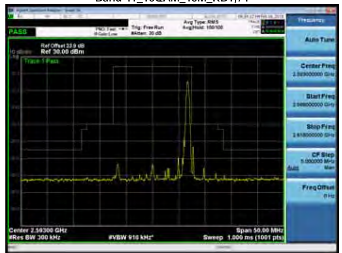
Band 41_16QAM_15M_RB1,74
