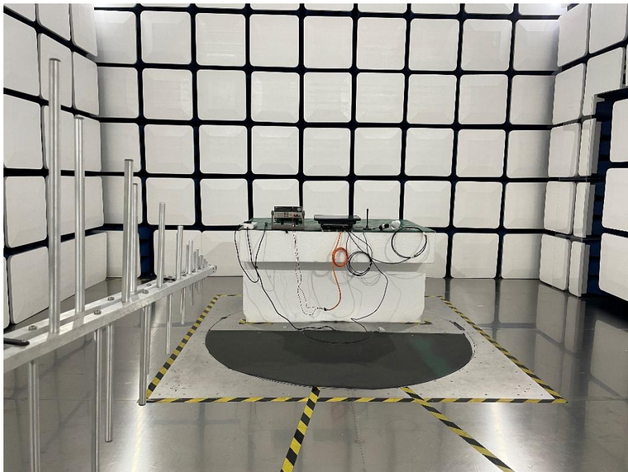
30 MHz-1 GHz-RF
