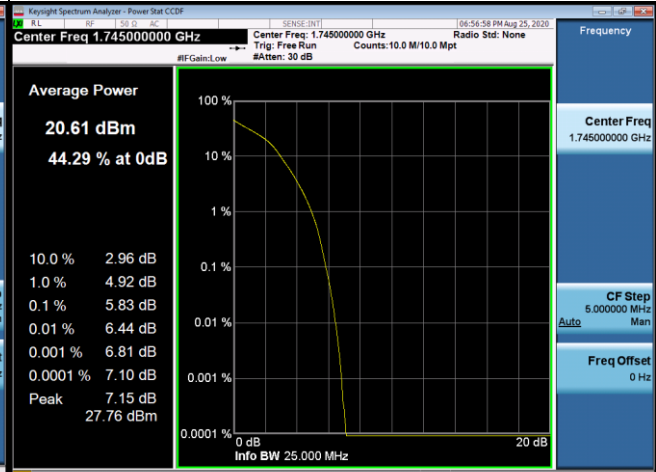
16QAM-20300
