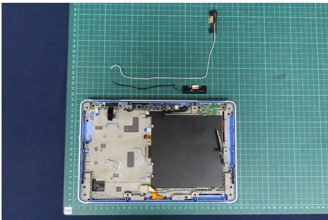
(19) EUT Photo
