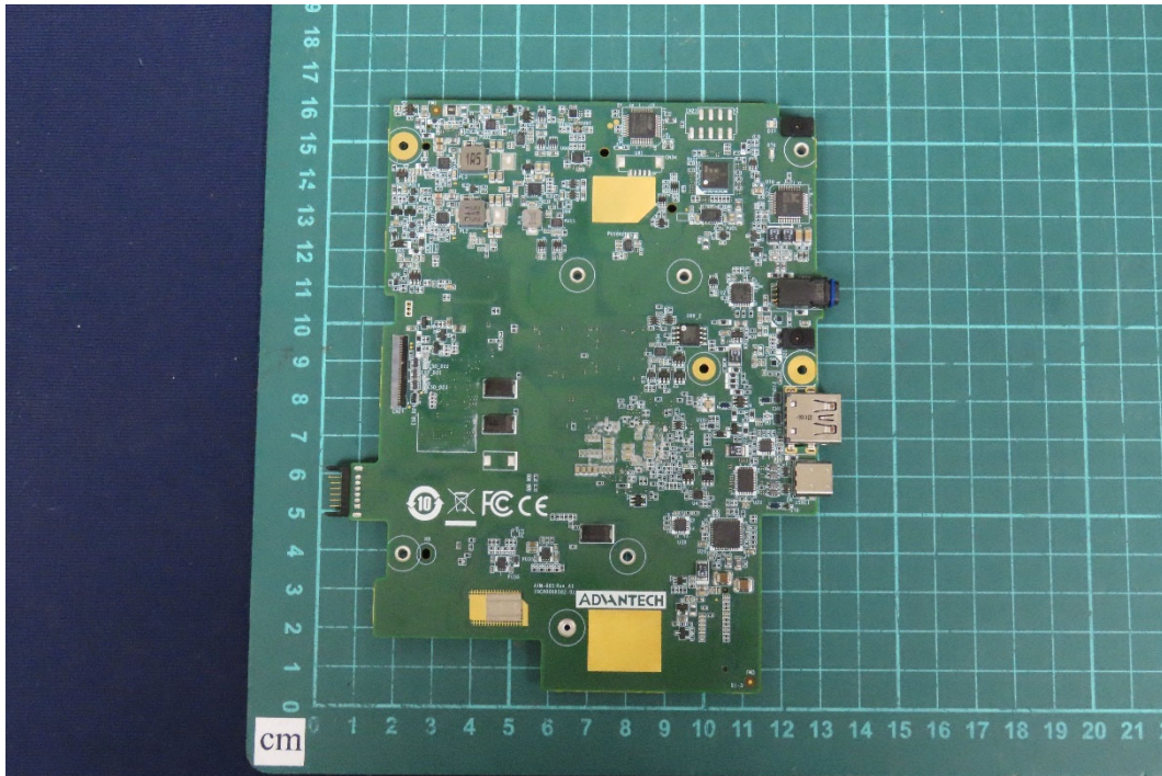
(17) EUT Photo
