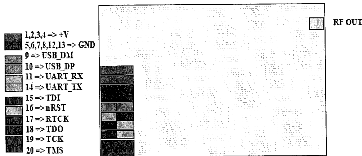
Fig 4-4. Pin Out for Handfree Mini Reader Module
