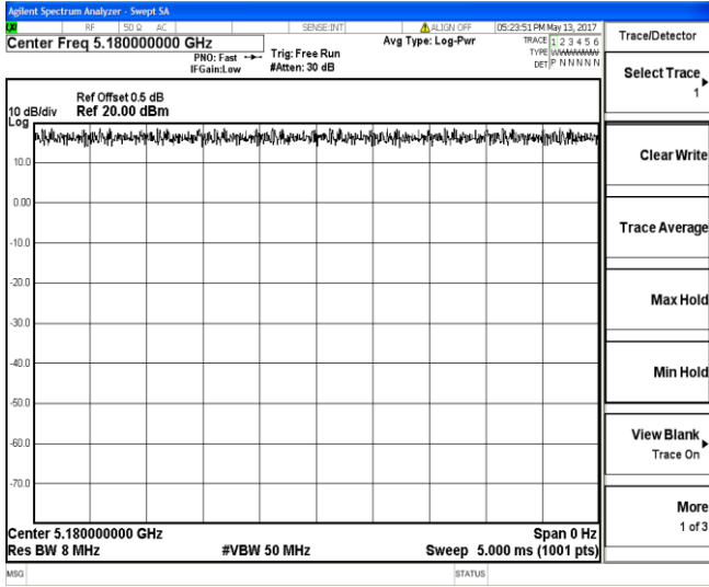
IEEE 802.11a
