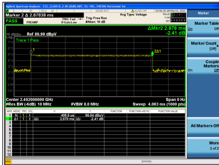
GFSK
