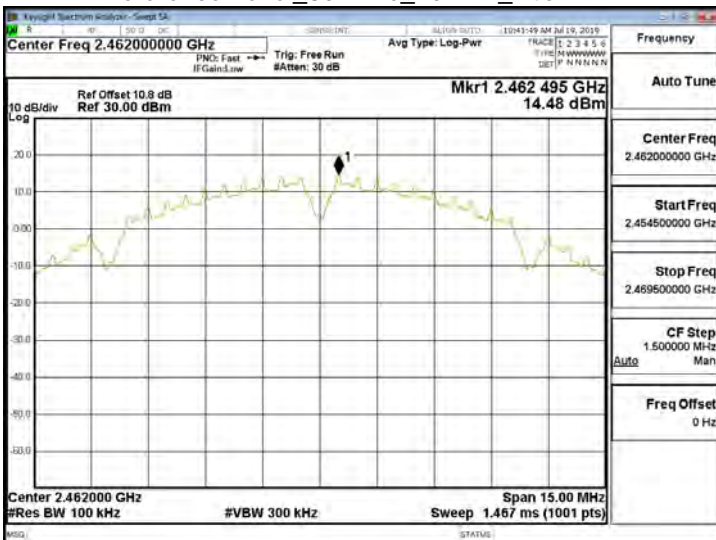
Reference Level_802.11b_20MHz_2462MHz
