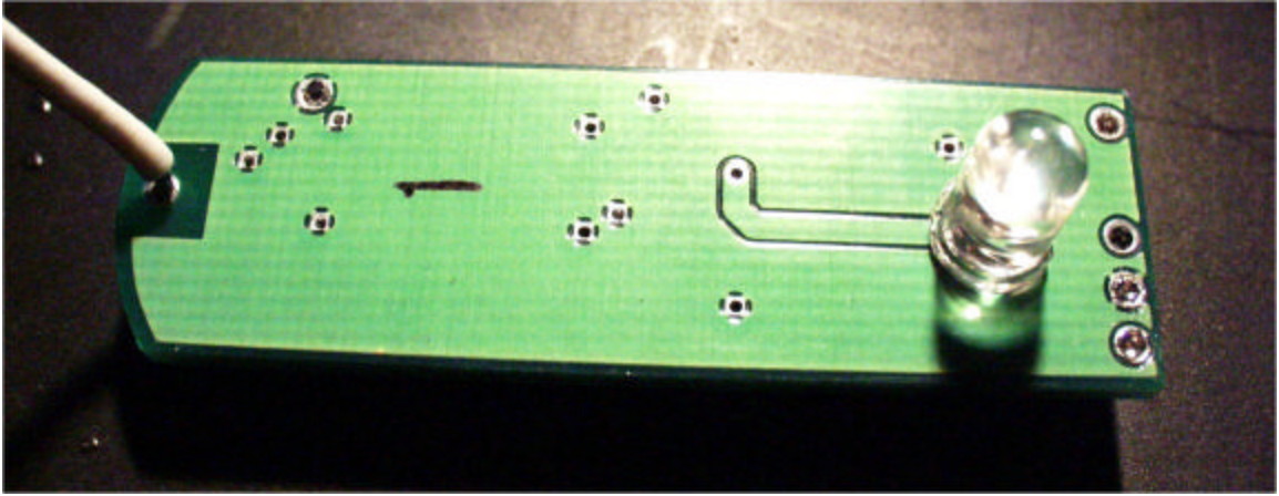
WRC TRANSMITTER PCA SOLDER SIDE.
