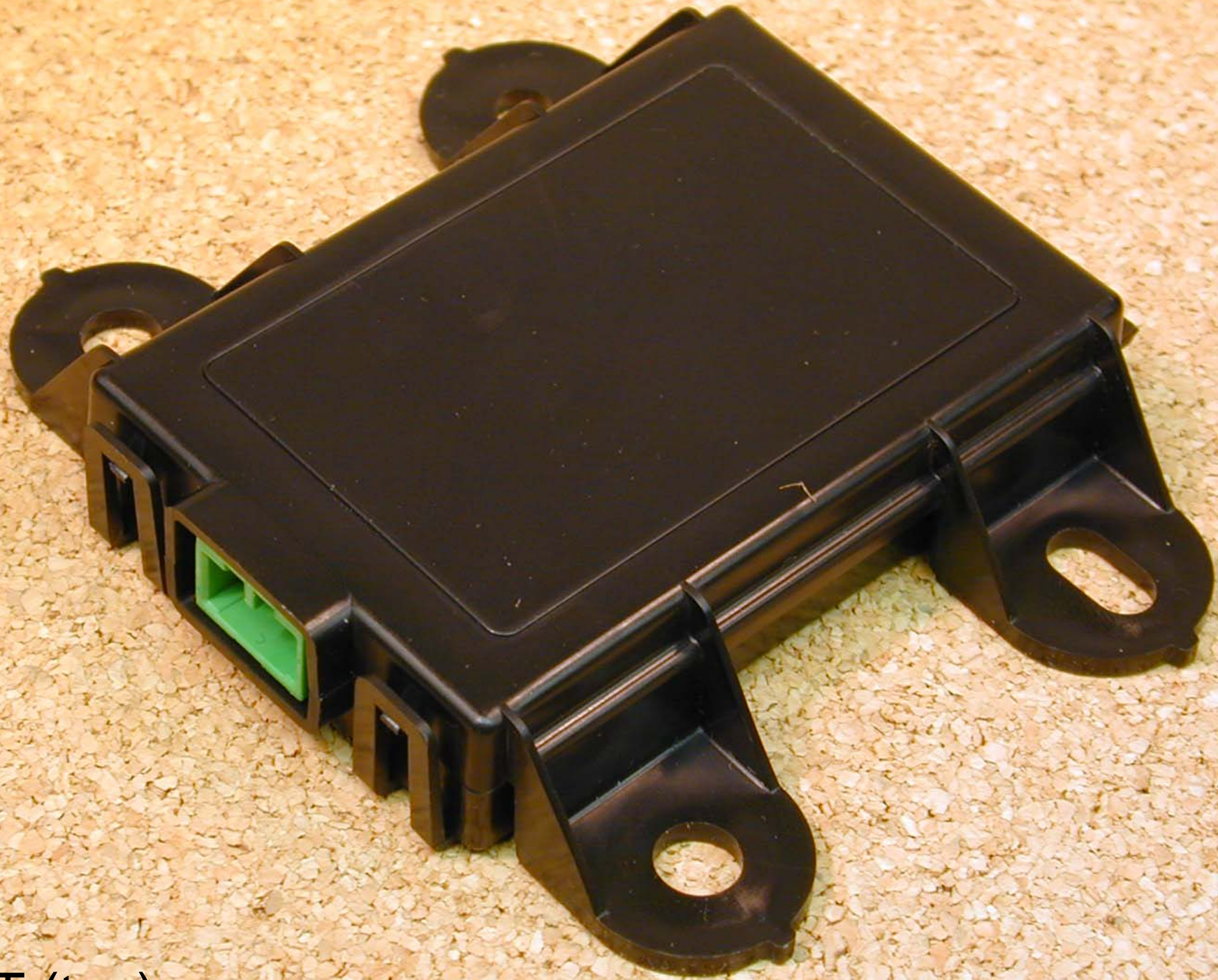
DUT (top)
