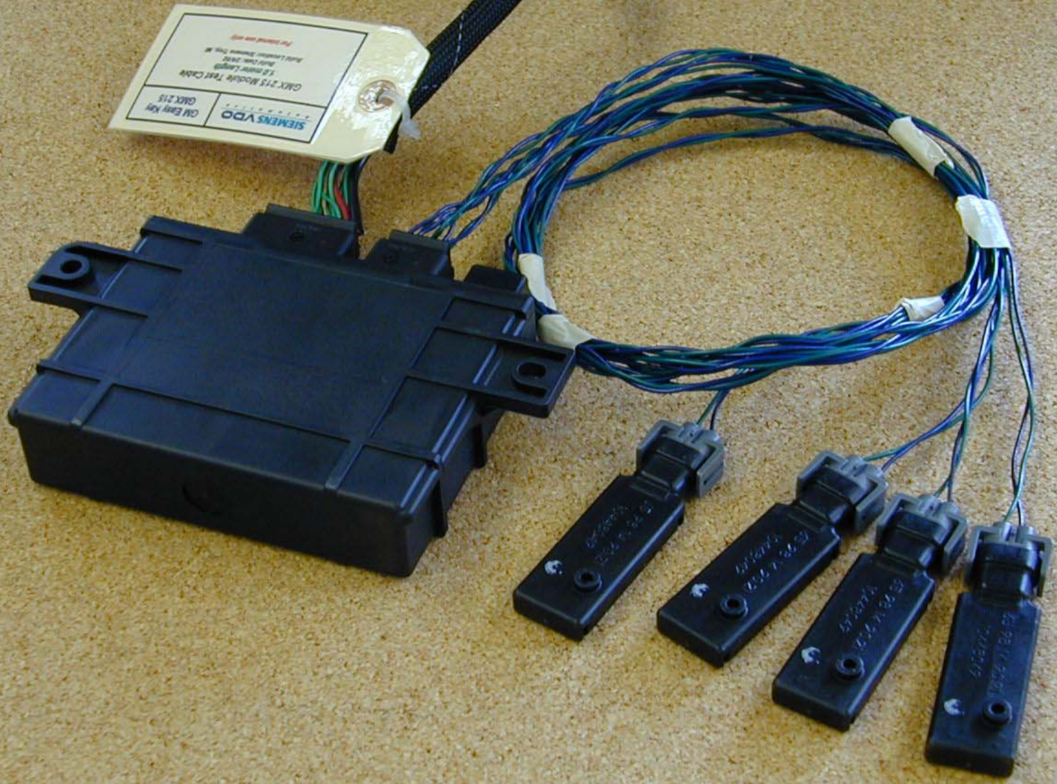
DUT (bottom)
