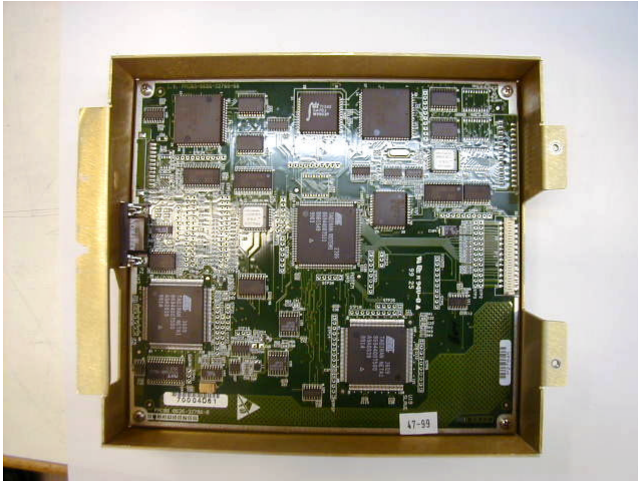
PRC-subassembly
