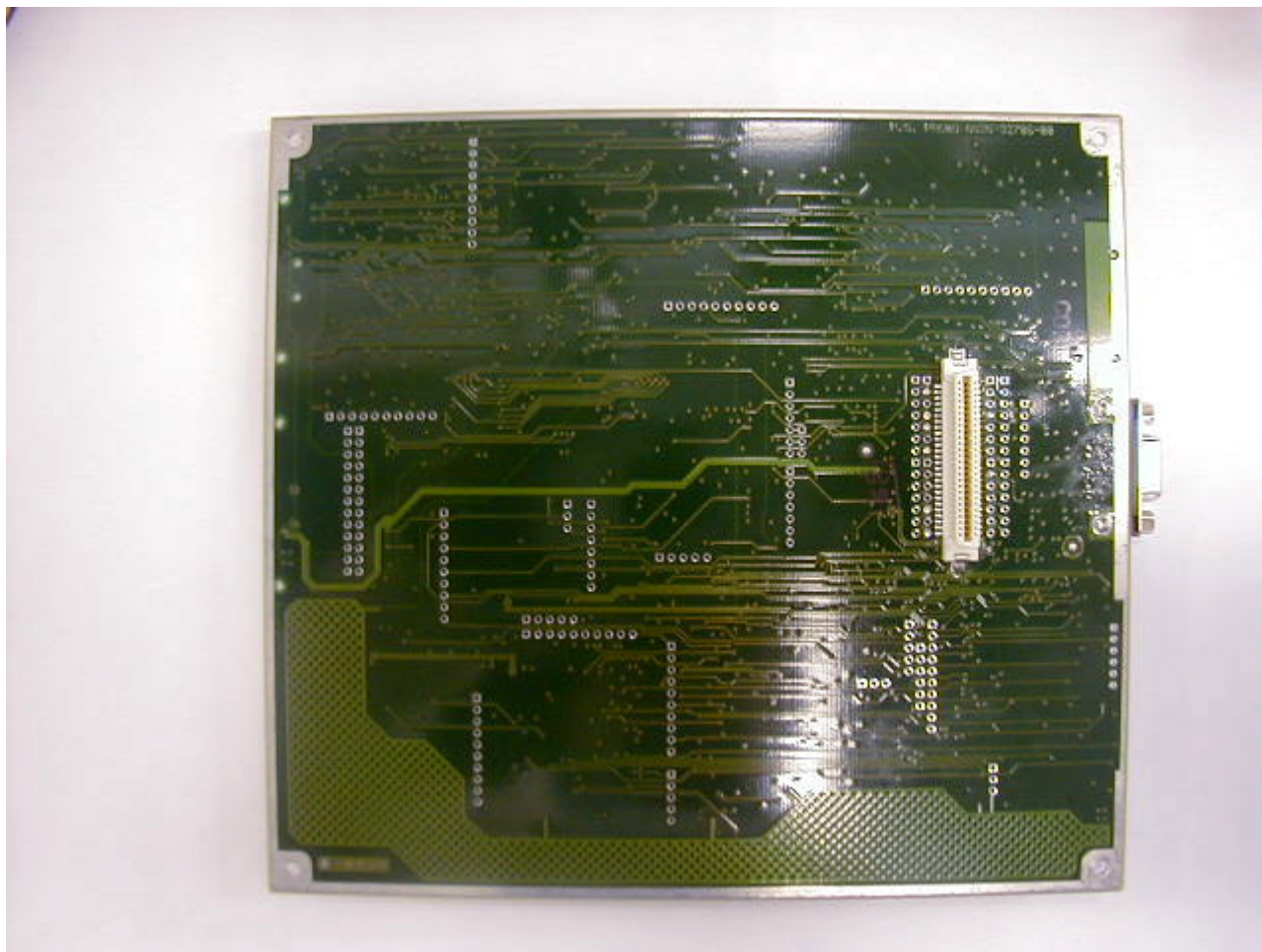
PRC-bottom
