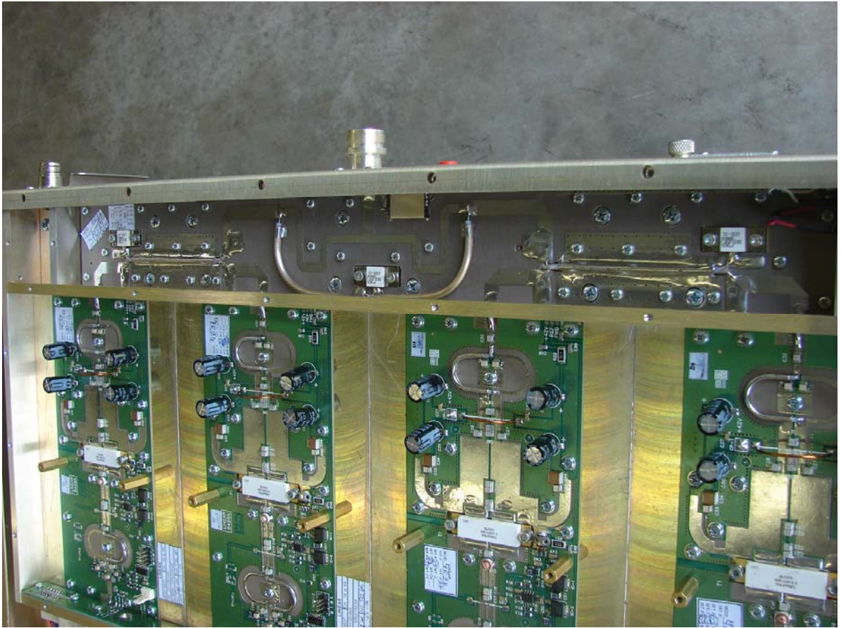
Output 4:1 Combiner
