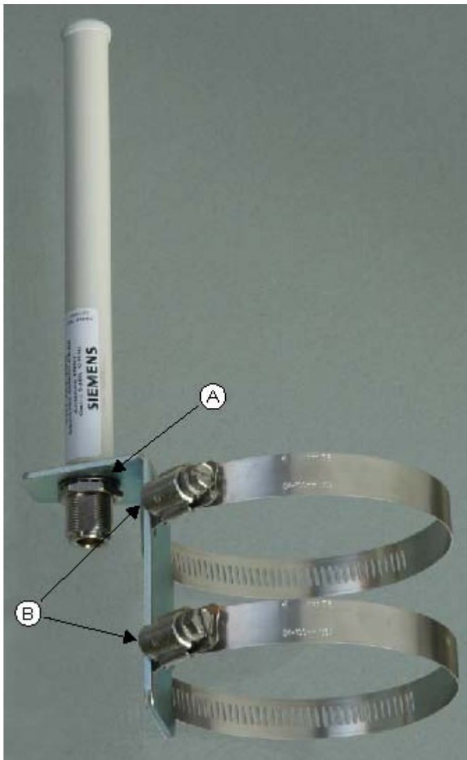
Abbildung 0-1 Montagemöglichkeit der ANT793-6MN - Mastmontage
