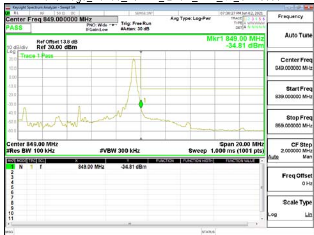
Band Edge_Band5_10MHz_QPSK_RB50_0_CH20450
