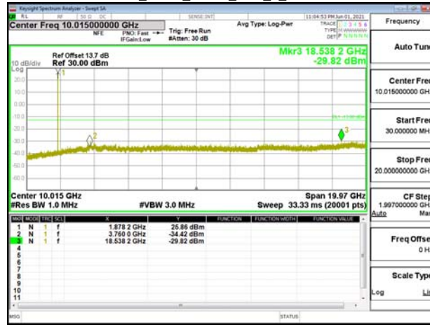
Band2_3MHz_QPSK_RB1_0_CH19185
