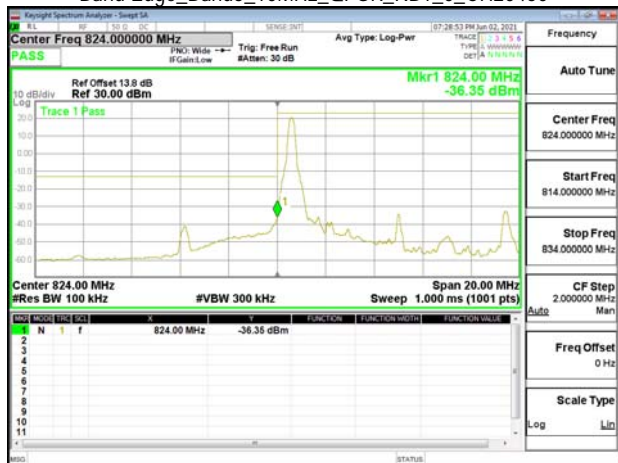
Band Edge_Band5_10MHz_QPSK_RB1_49_CH20600
