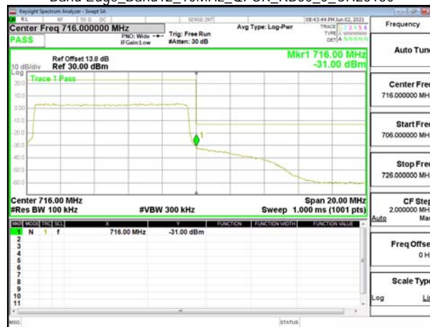
Band Edge_Band12_10MHz_QPSK_RB50_0_CH23130
