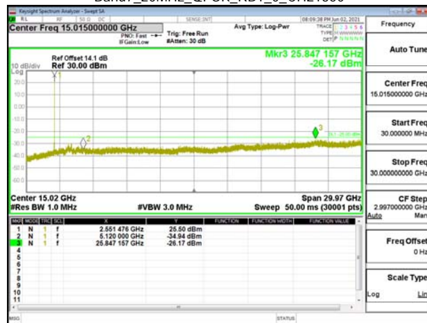
Band7_20MHz_QPSK_RB1_0_CH21350
