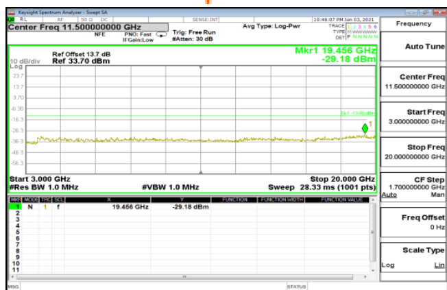
GPRES_1900MHz_MidCH661-1880
