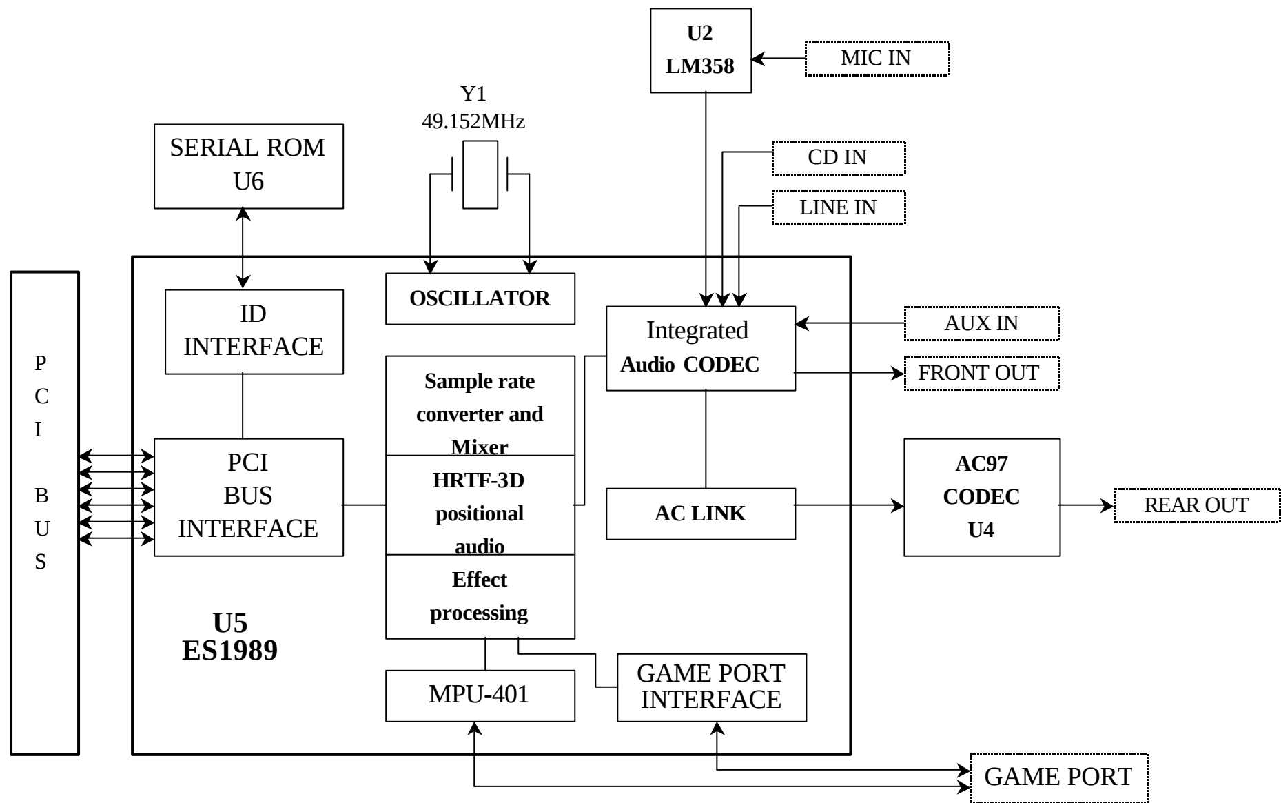
A571-T20 BLOCK DIAGRAM
