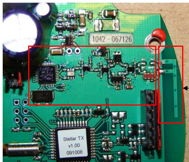
Antenna
