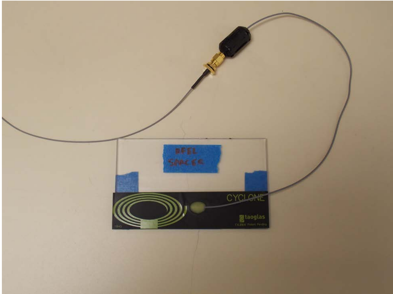
WWAN Antenna
