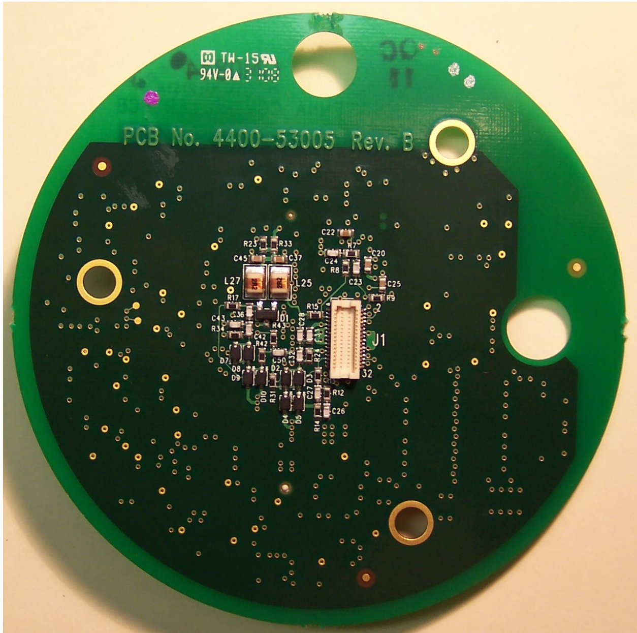
Top PCB
