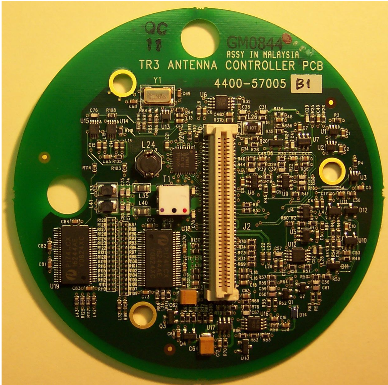
Bottom PCB
