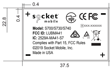
SCALE 2:1
