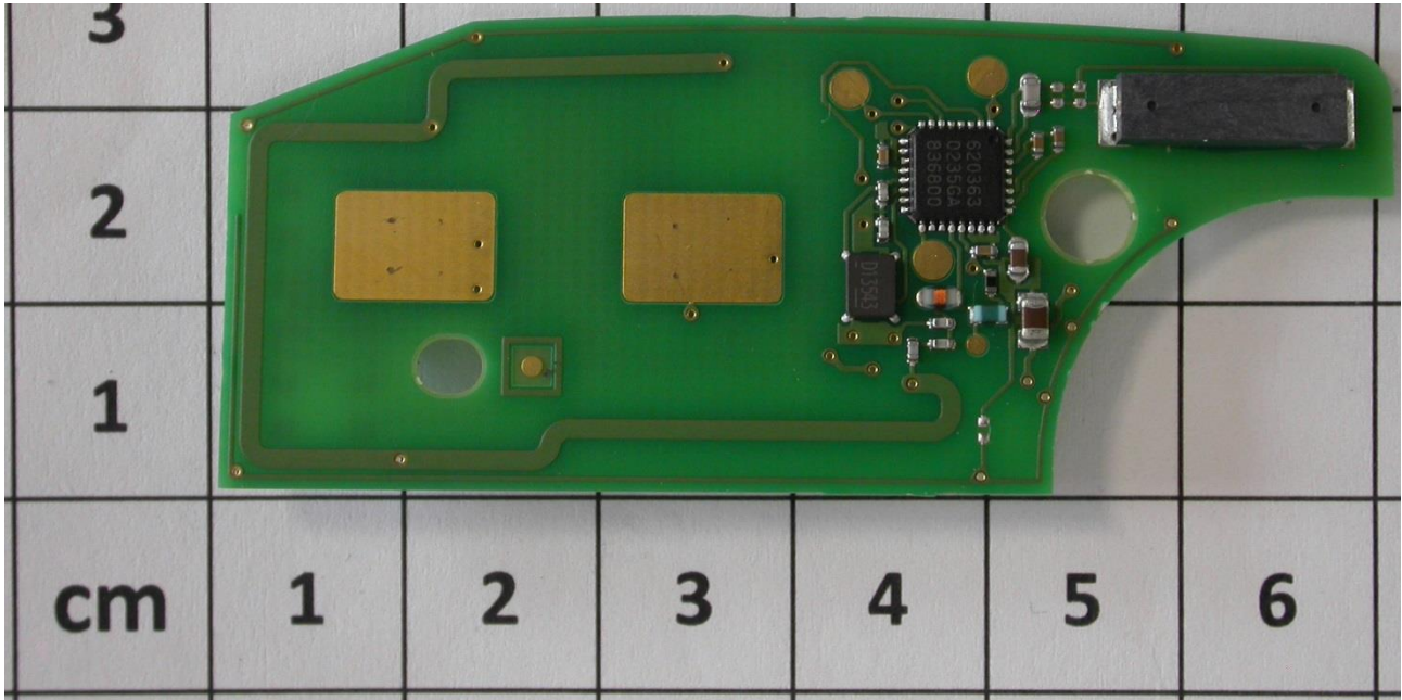
PCB bottom
